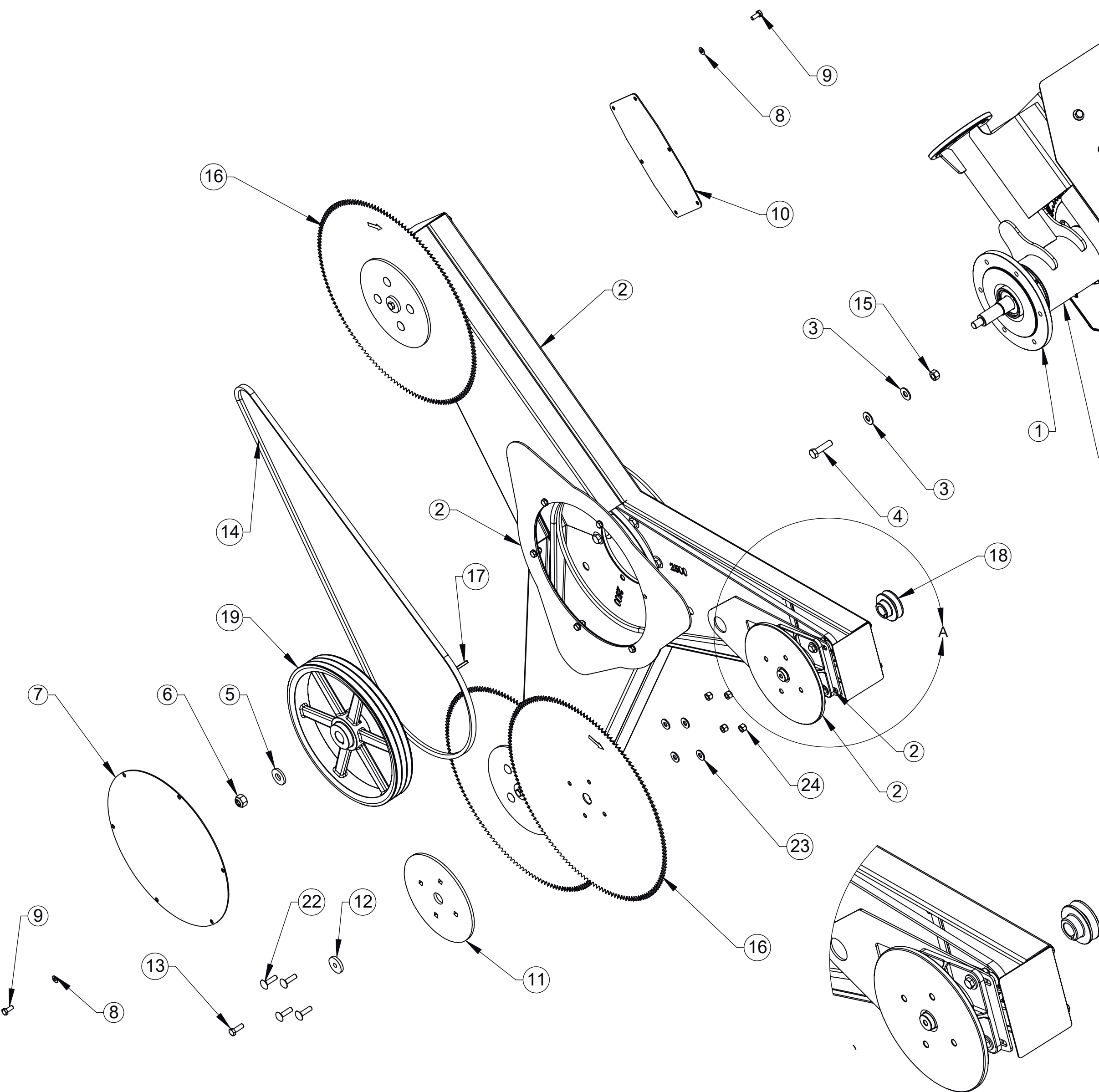
DETALHE A DA POLIA CANAL B ESCALA 1 : 7
