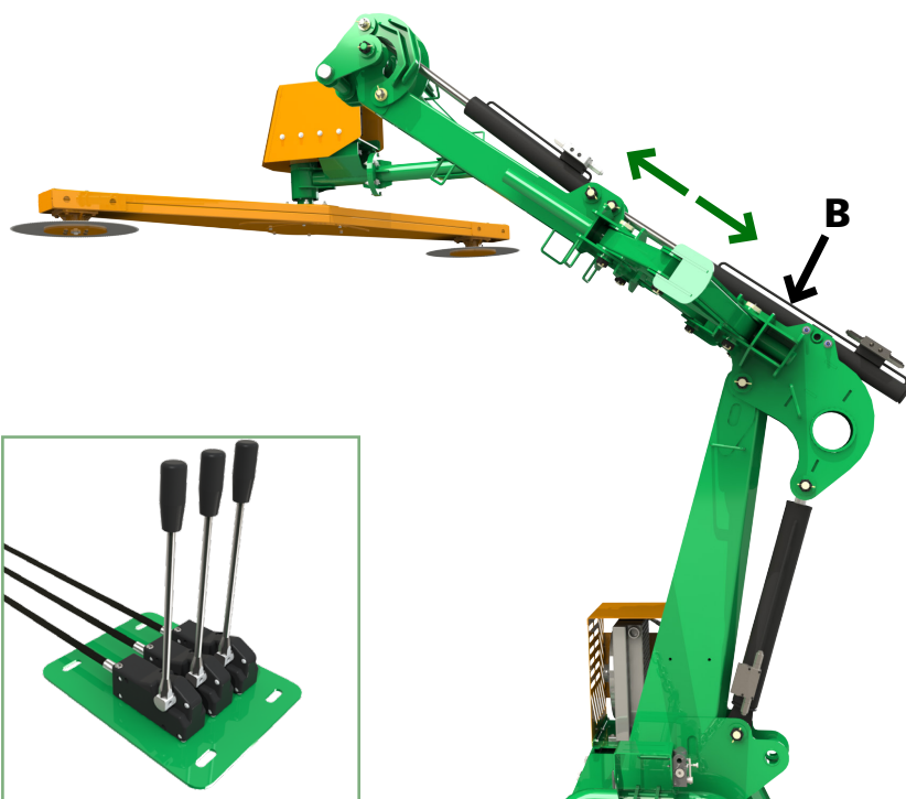
comando hidráulico
