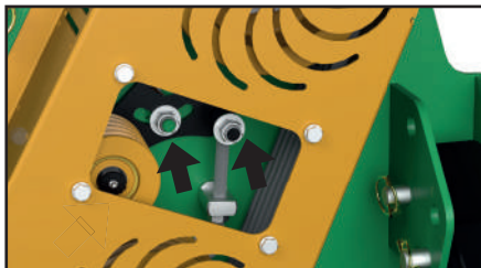
Retirar a tampa e lubrificar o rolete do esticador
