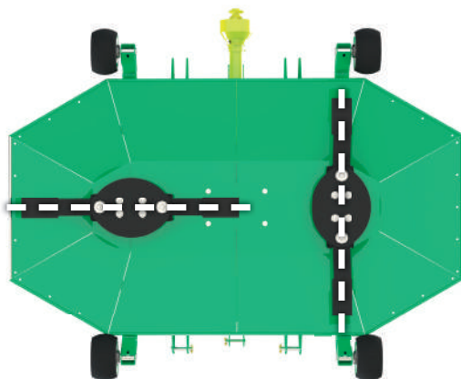
REGULAGEM CORRETA DOS ROTORES
