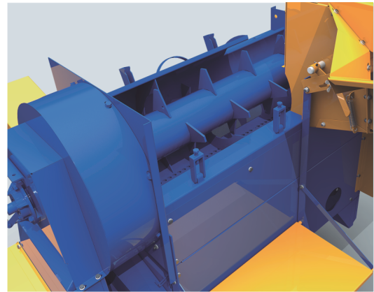
Potente rotor procesa el cereal sin dañar los granos.
